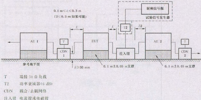
其他连接线
