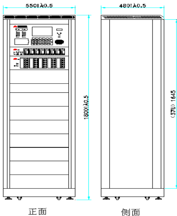
JB-TG-JF999 火灾报警控制器消防联动控制器外形图：
