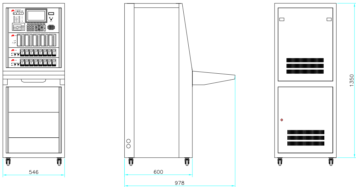
JB-TT-JF999 火灾报警控制器消防联动控制器外形图：
