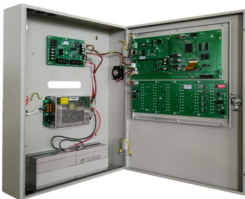
图 4 JF-FH1000 内部结构
