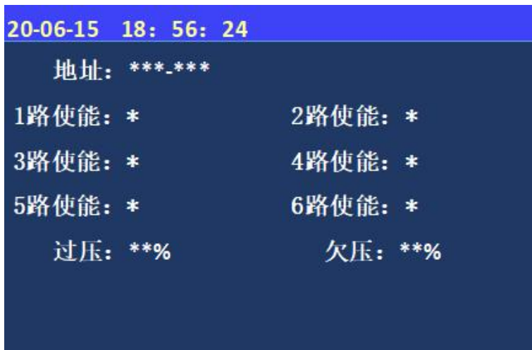
图 5-3-6 设置单相电压参数
