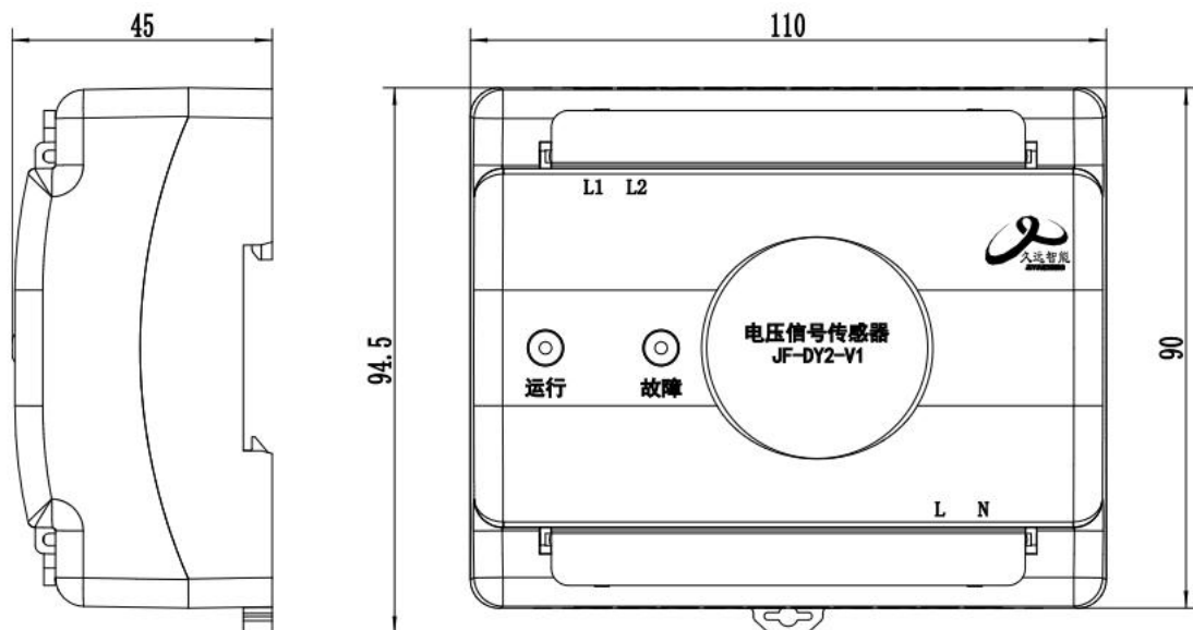
图 1 外形尺寸图
