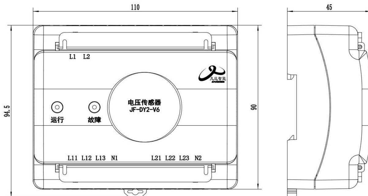
图 1 外形尺寸图
