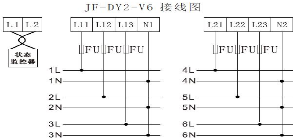
图 2 接线示意图
