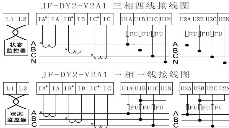
图 2 接线示意图
