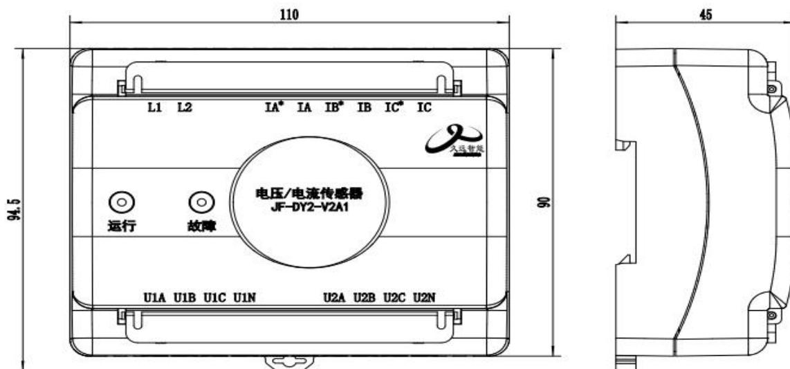
图 1 外形尺寸图
