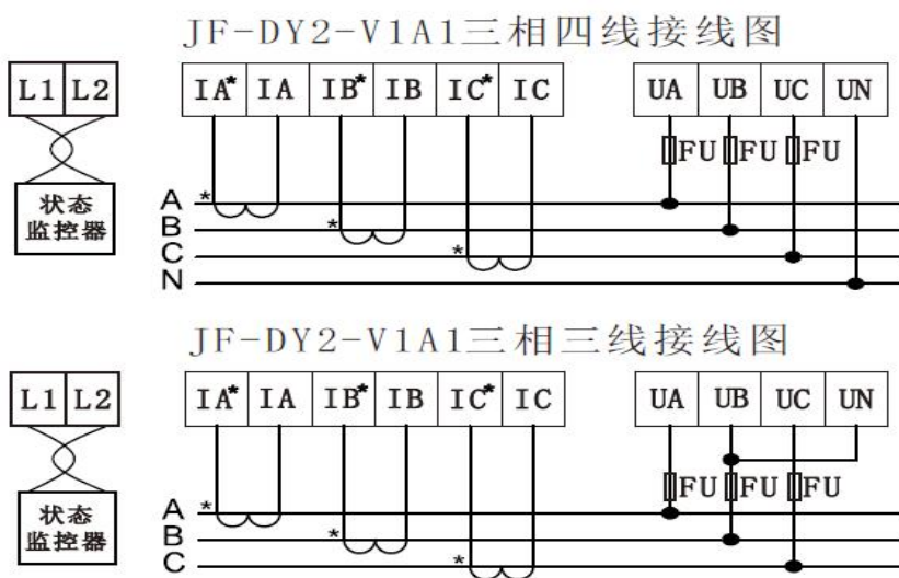
图 2 接线示意图
