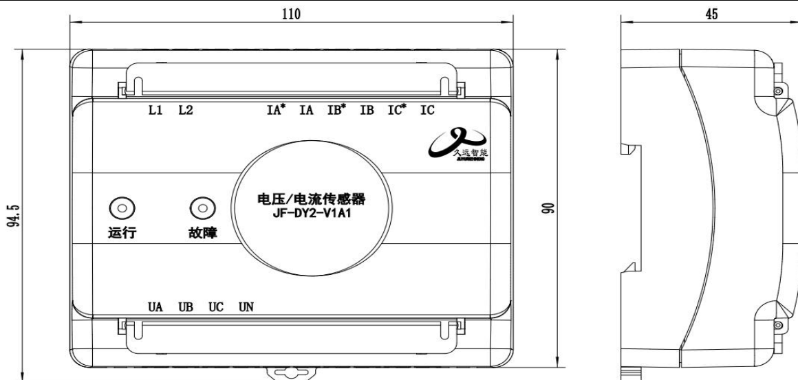
图 1 外形尺寸图
