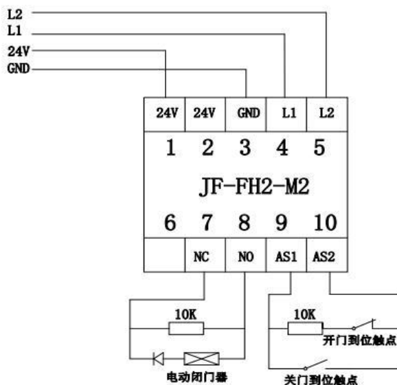
图 4 接线示意图
