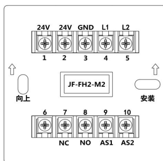
图 2 端子图
