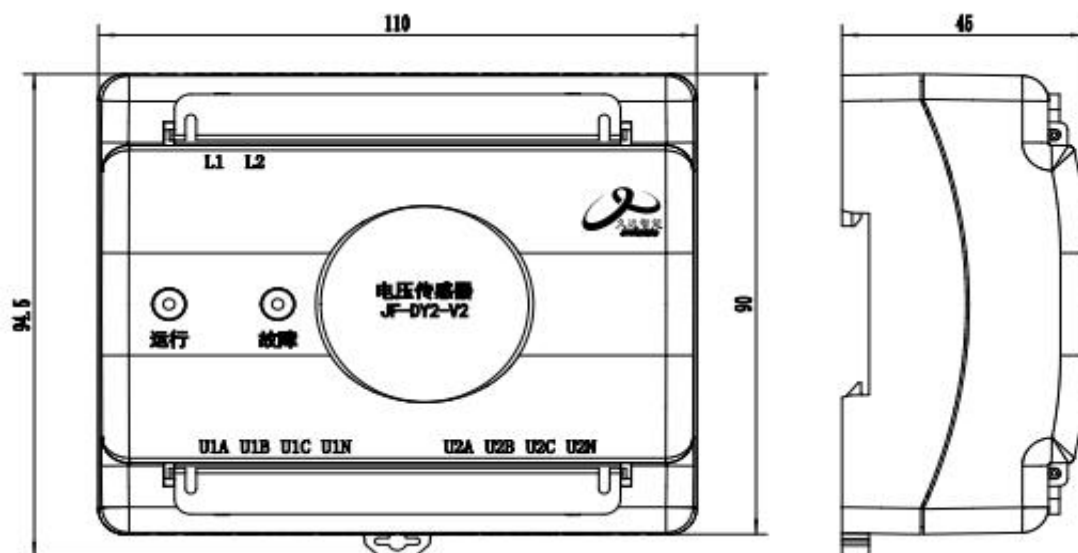
图 1 外形尺寸图
