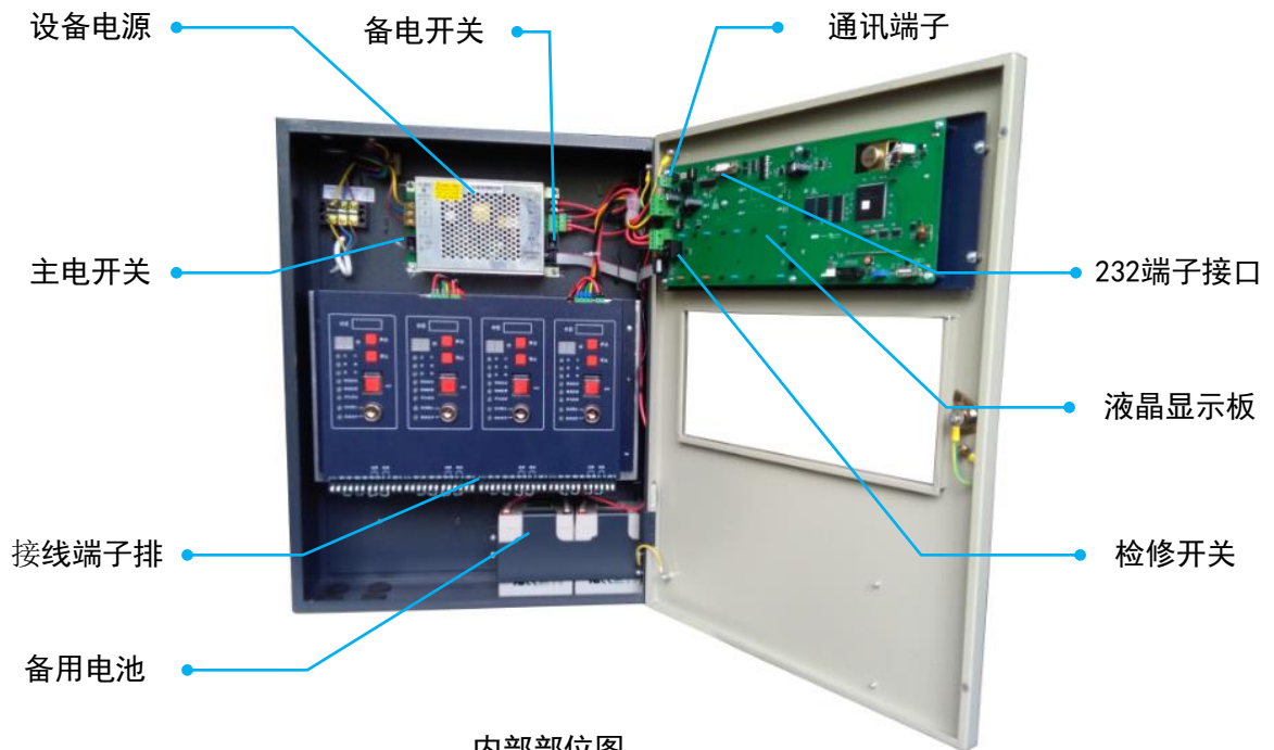
内部部位图
