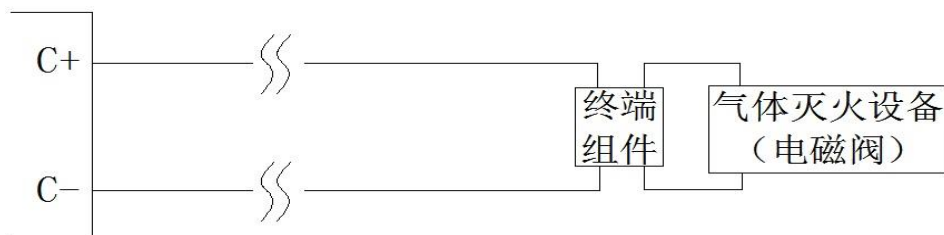
图 1 喷洒启动输出接线示意图（连接电磁阀式气灭设备）
