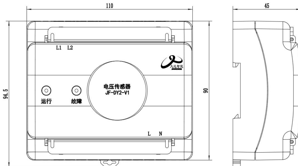
图 1 外形尺寸图
