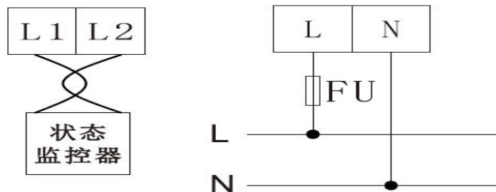
JF-DY2-V1 接线图
